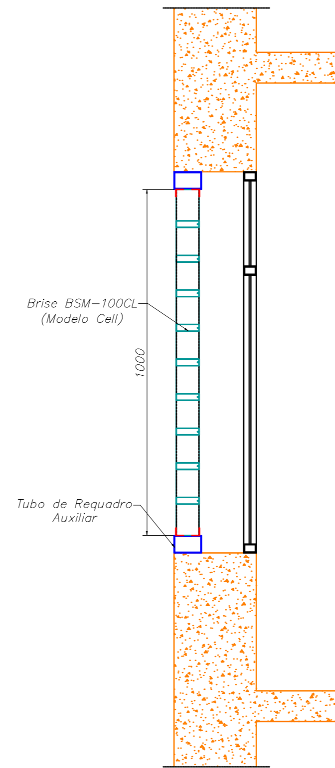
BRISES BSM-100CL DENTRO DO VÃO ESCALA: 1:10
