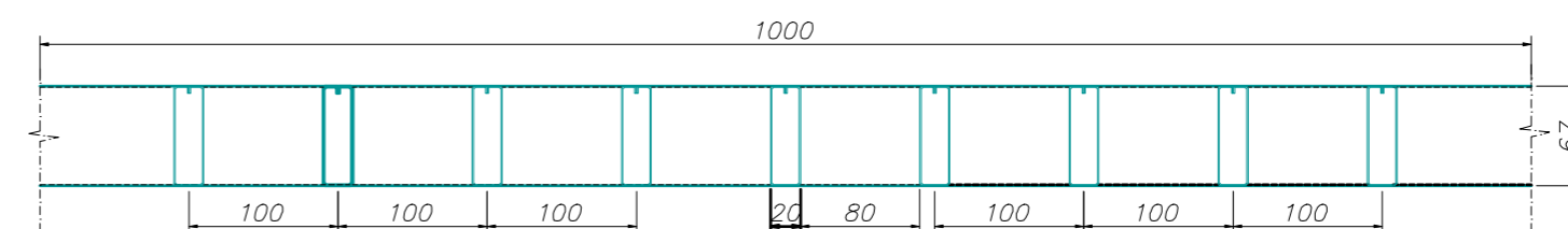
DETALHE DA MALHA DO BRISE BSM-100CL Escala: 1:5
