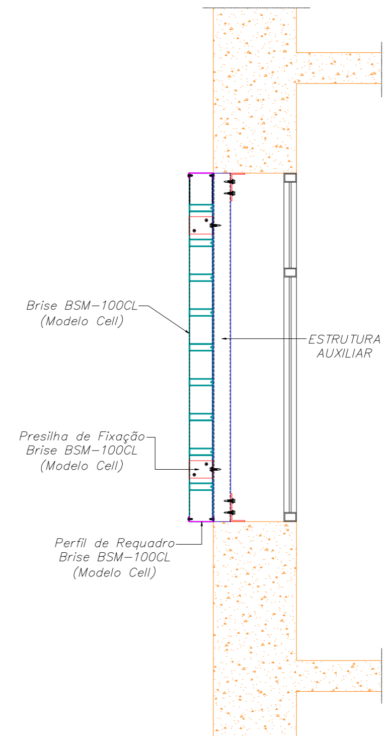
BRISES BSM-100CL FORA DO VÃO ESTRUTURA OCLUSA ESCALA: 1:10
