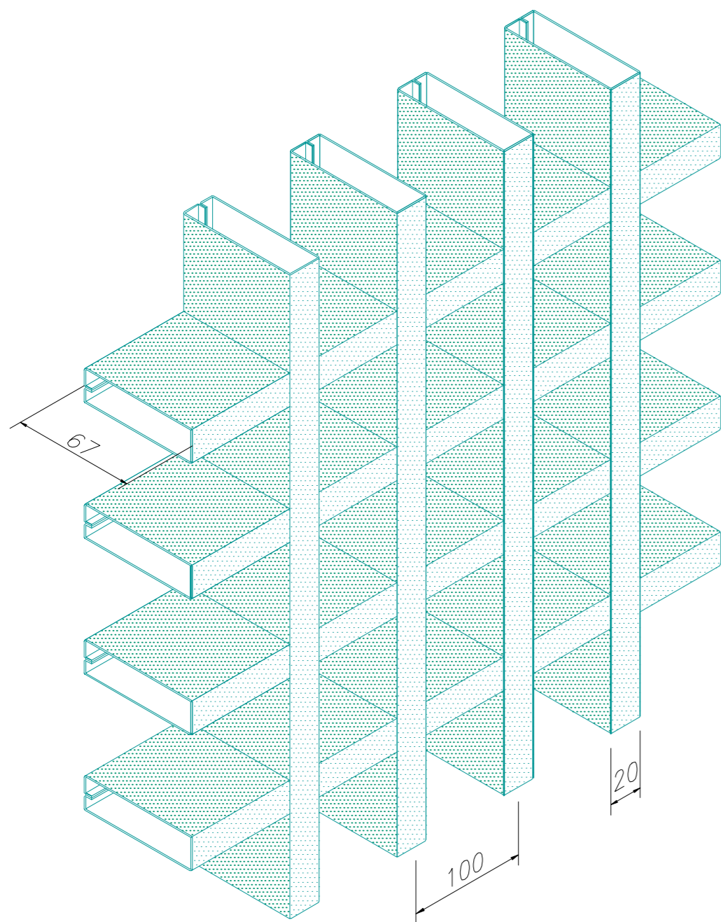
PERSPECTIVA ILUSTRATIVA BSM-100CL Escala: S/E
