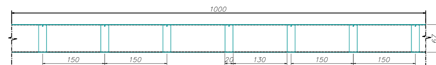
DETALHE DA MALHA DO BRISE BSM-150CL Escala: 1:5
