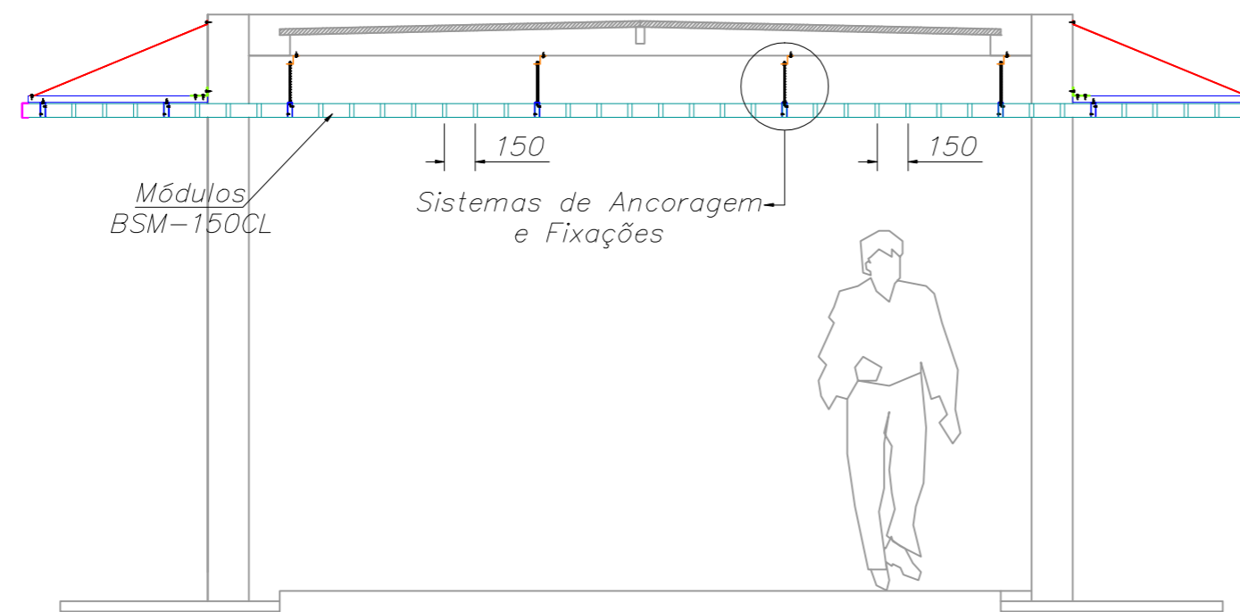
DETALHE DE APLICAÇÃO DO BSM-150CL COMO FORRO Escala: 1:30
