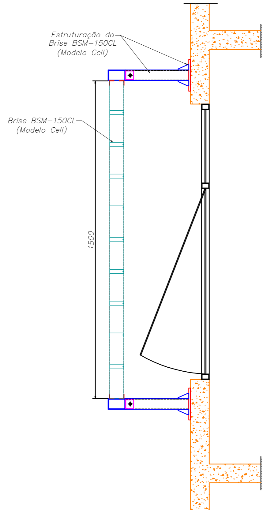
BRISES BSM-150CL FORA DO VÃO ESCALA: 1:10
