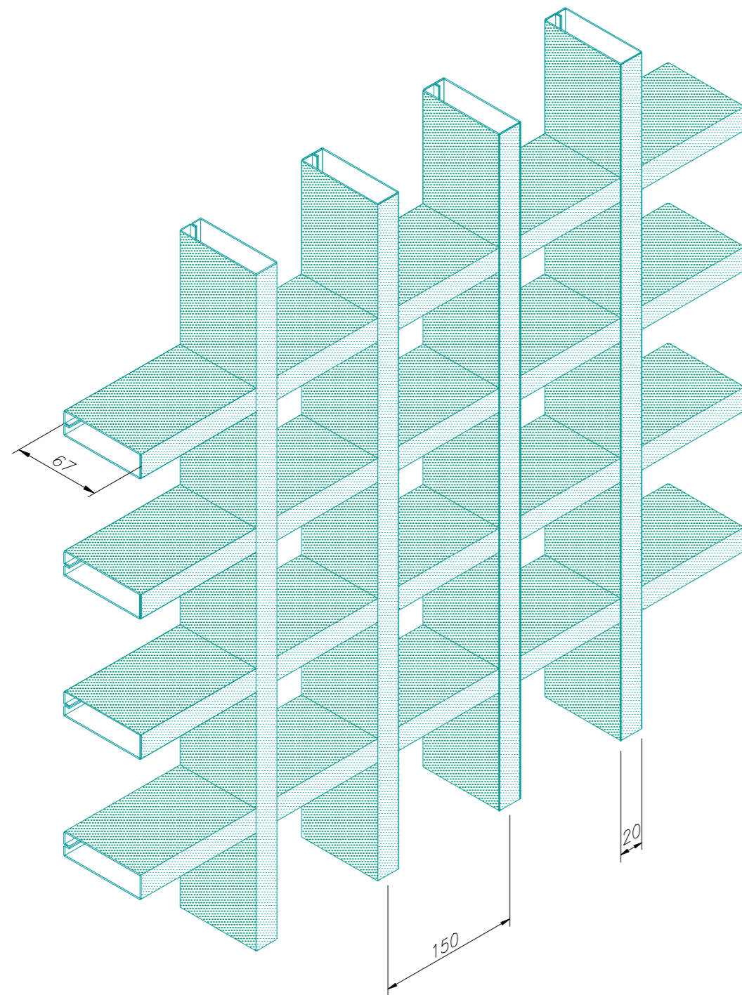
PERSPECTIVA ILUSTRATIVA BSM-150CL Escala: S/E
