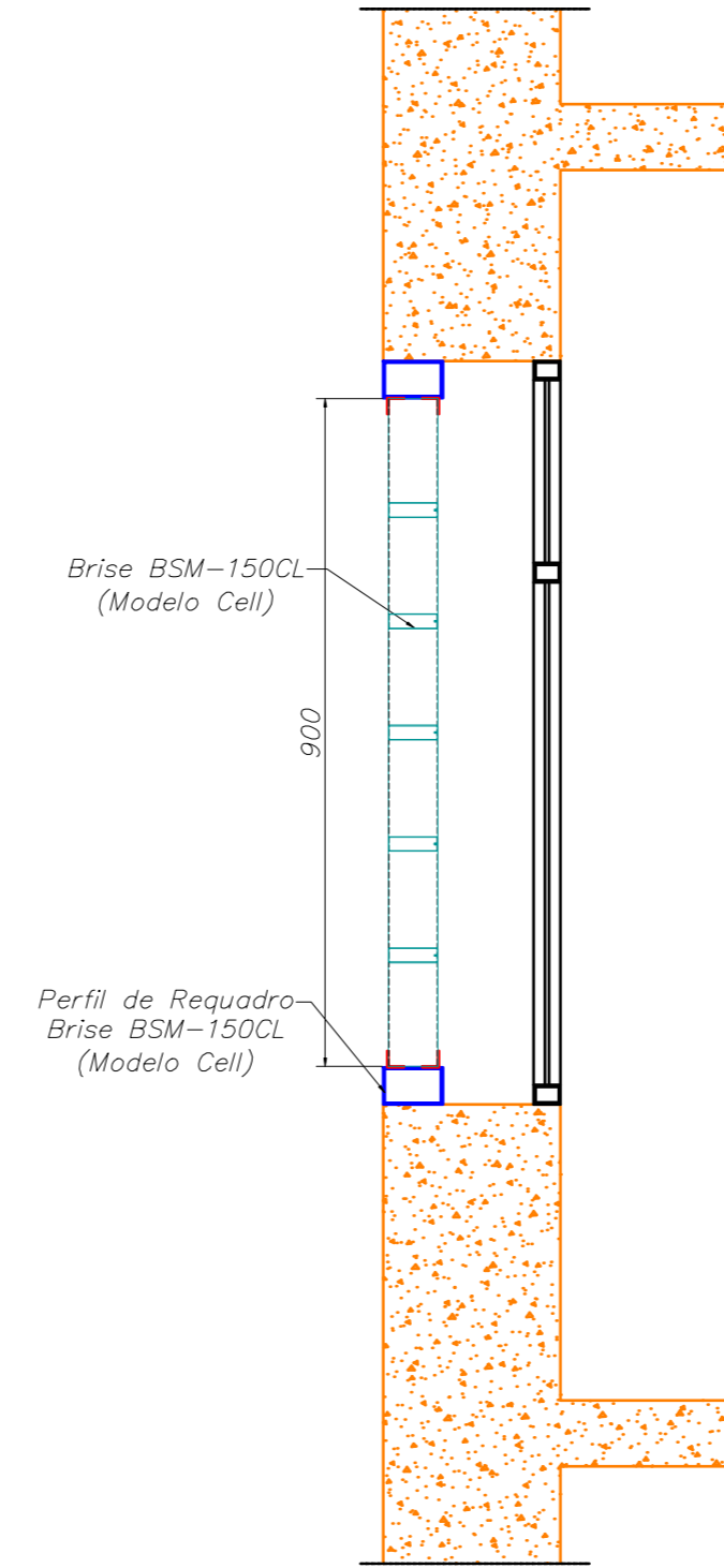
BRISES BSM-100CL DENTRO DO VÃO ESCALA: 1:10
