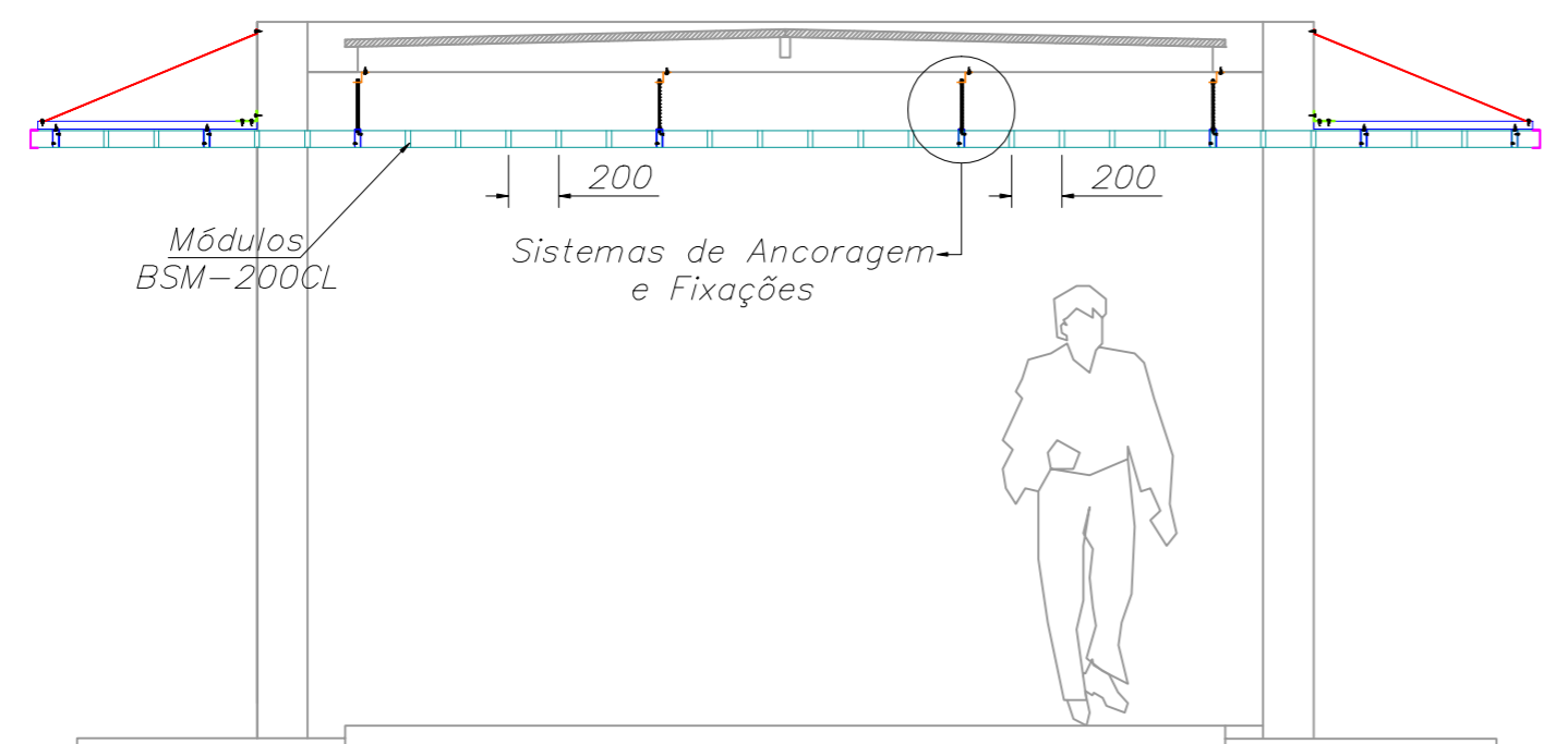
DETALHE DE APLICAÇÃO DO BSM-200CL COMO FORRO Escala: 1:30
