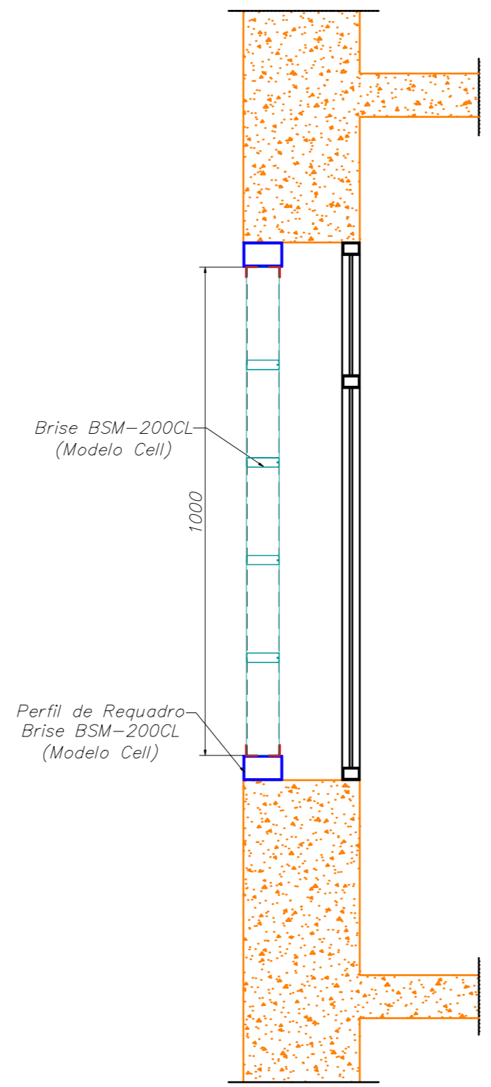
BRISES BSM-100CL DENTRO DO VÃO ESCALA: 1:10
