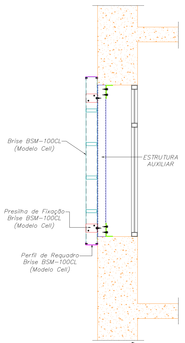
BRISES BSM-100CL FORA DO VÃO ESTRUTURA OCLUSA ESCALA: 1:10
