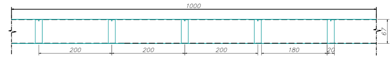
DETALHE DA MALHA DO BRISE BSM-200CL Escala: 1:5
