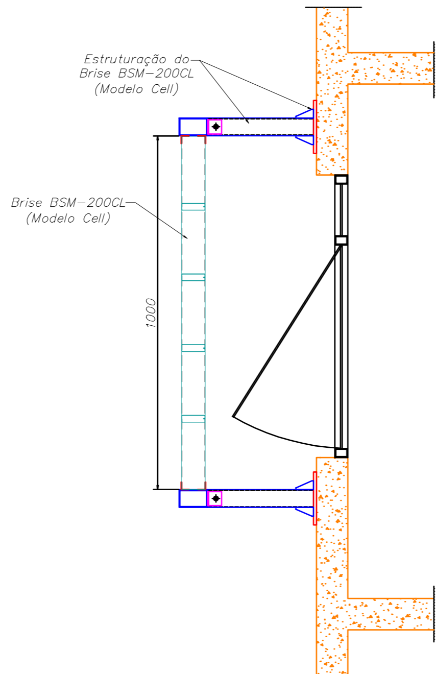
BRISES BSM-100CL FORA DO VÃO ESCALA: 1:10
