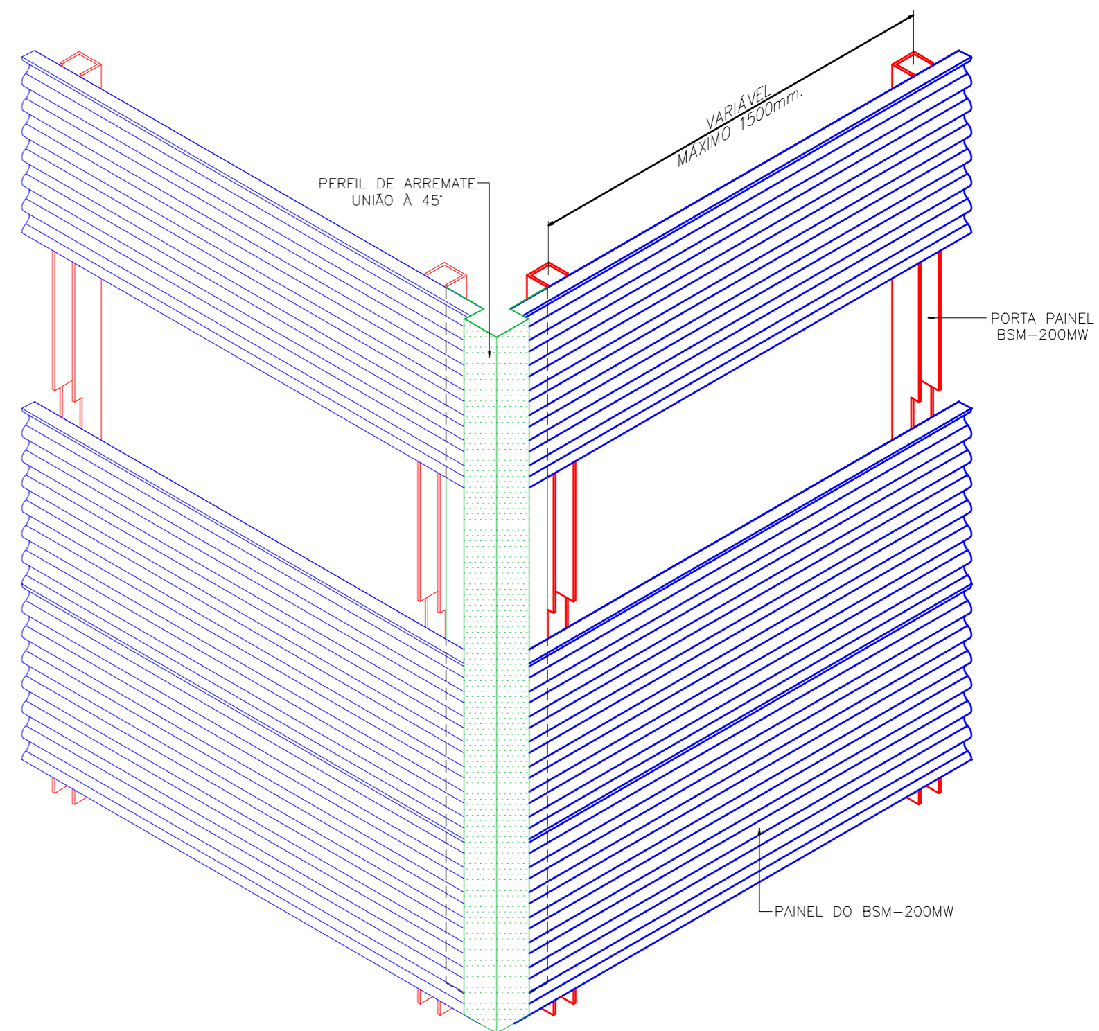
PERSPECTIVA DO BSM-200MW ENCONTRO À 45°
