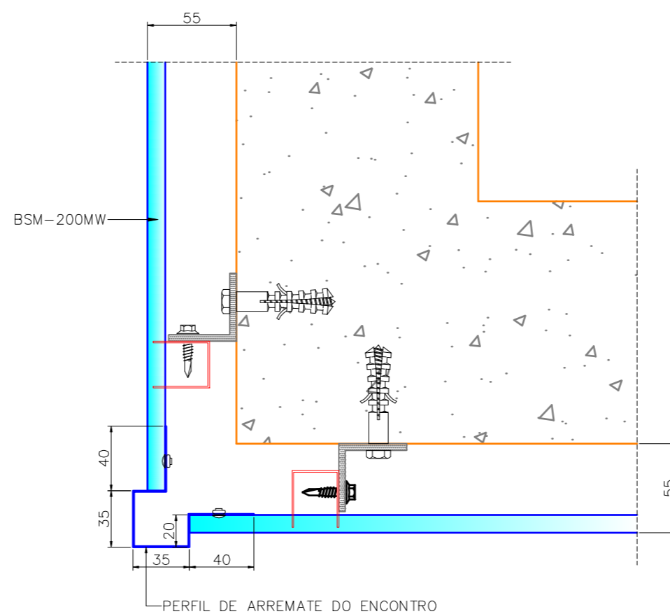
DETALHE DO ENCONTRO DAS LÂMINAS
