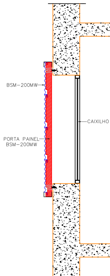
BRISE BSM-200MW FORA DO VÃO
