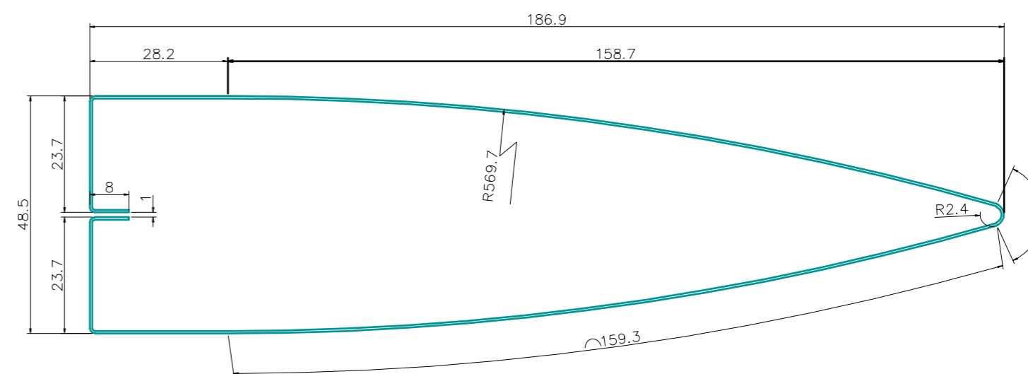
DETALHE DA LÂMINA DO BSM-A200
