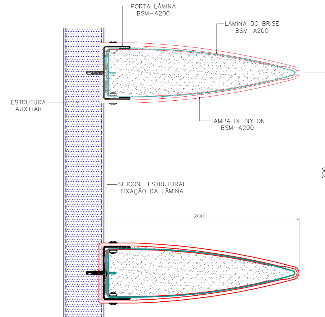
DETALHE DE FIXAÇÃO DO BSM-A200
