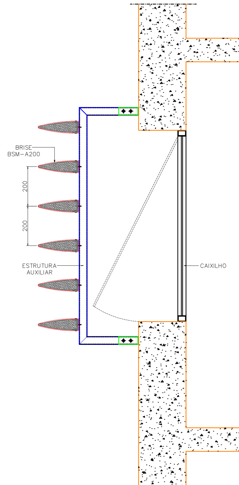
BRISE BSM-A100 FORA DO VÃO
