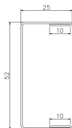
PORTA LÂMINA DO BSM-A200
