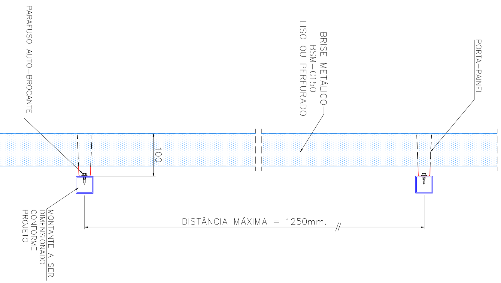
CORTE "AA"
