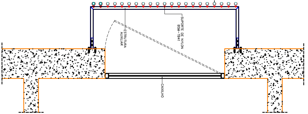
BRISE BSM-TB41 FORA DO VÃO
