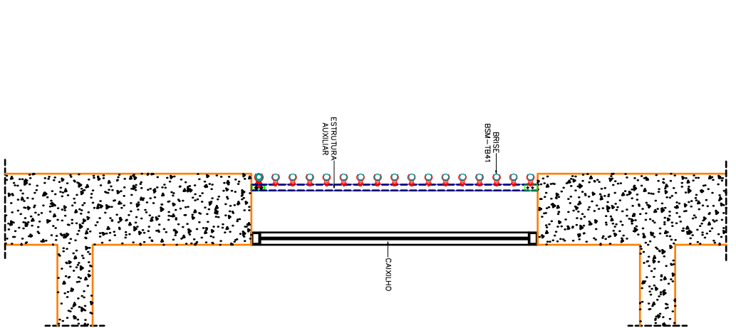
BRISE BSM-TB41 DENTRO DO VÃO
