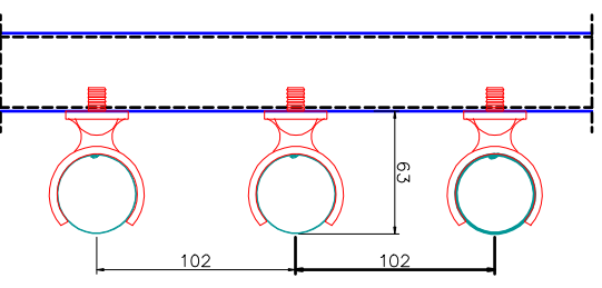
DETAILHE BSM-TB41 - PASSO DE 102mm.
