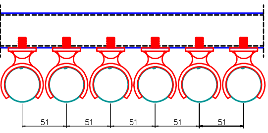
DETAILHE BSM-TB41 - PASSO DE 51mm.
