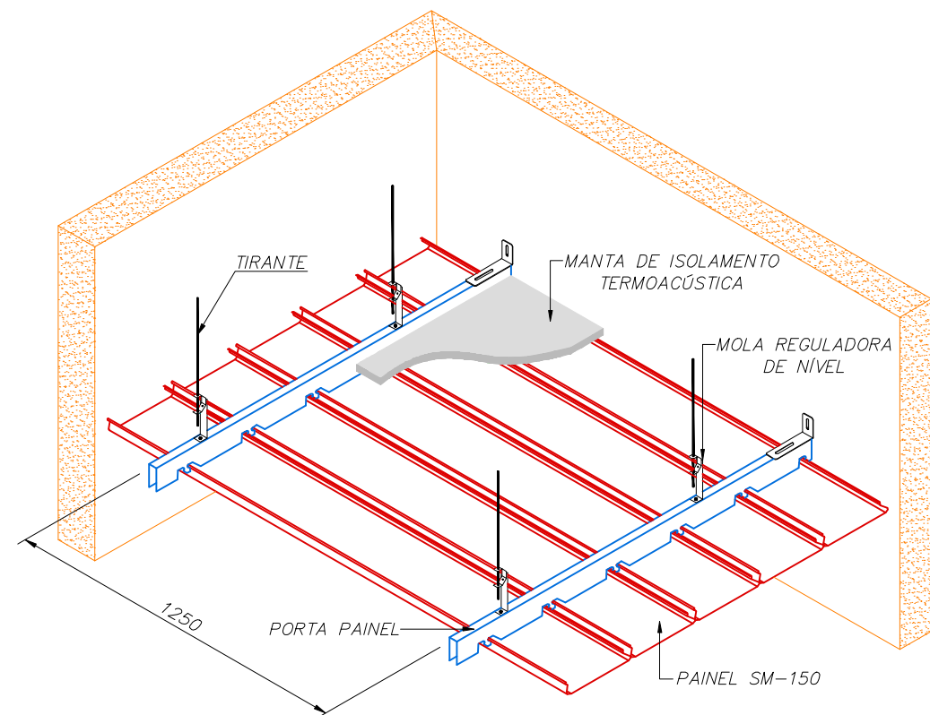
ESQUEMA DE MONTAGEM FORRO SM-150 Escala: 1:2
