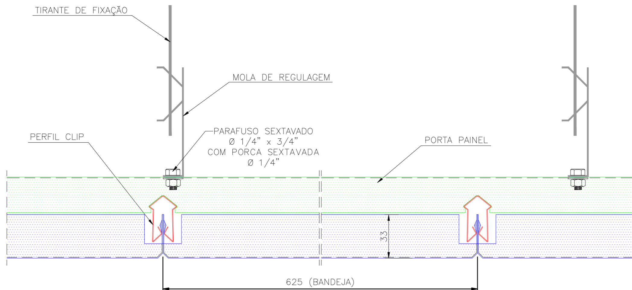
DETALHE DE JUNÇÃO DO FORRO SM-625CI SENTIDO LONGITUDINAL
