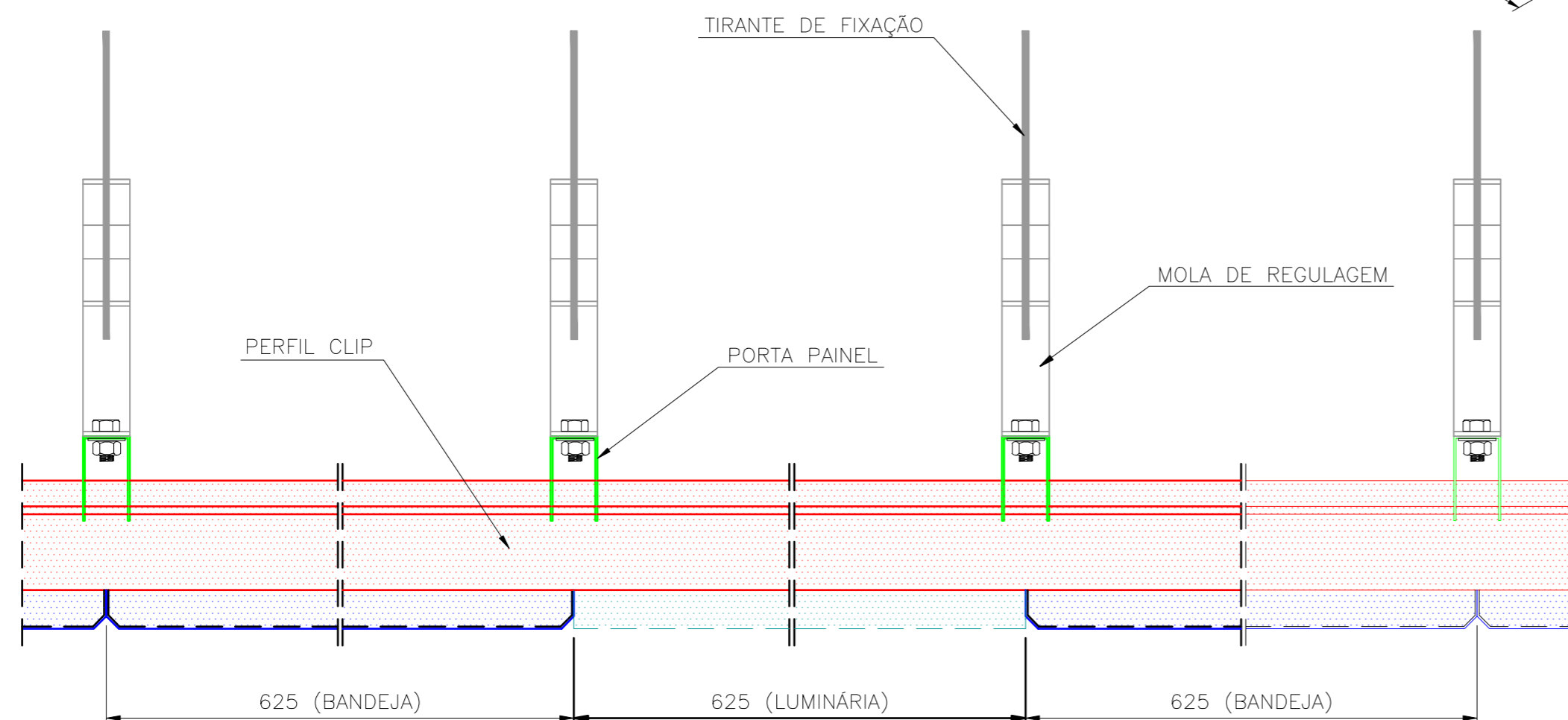
DETALHE DE JUNÇÃO DO FORRO SM-625CI SENTIDO TRANSVERSAL
