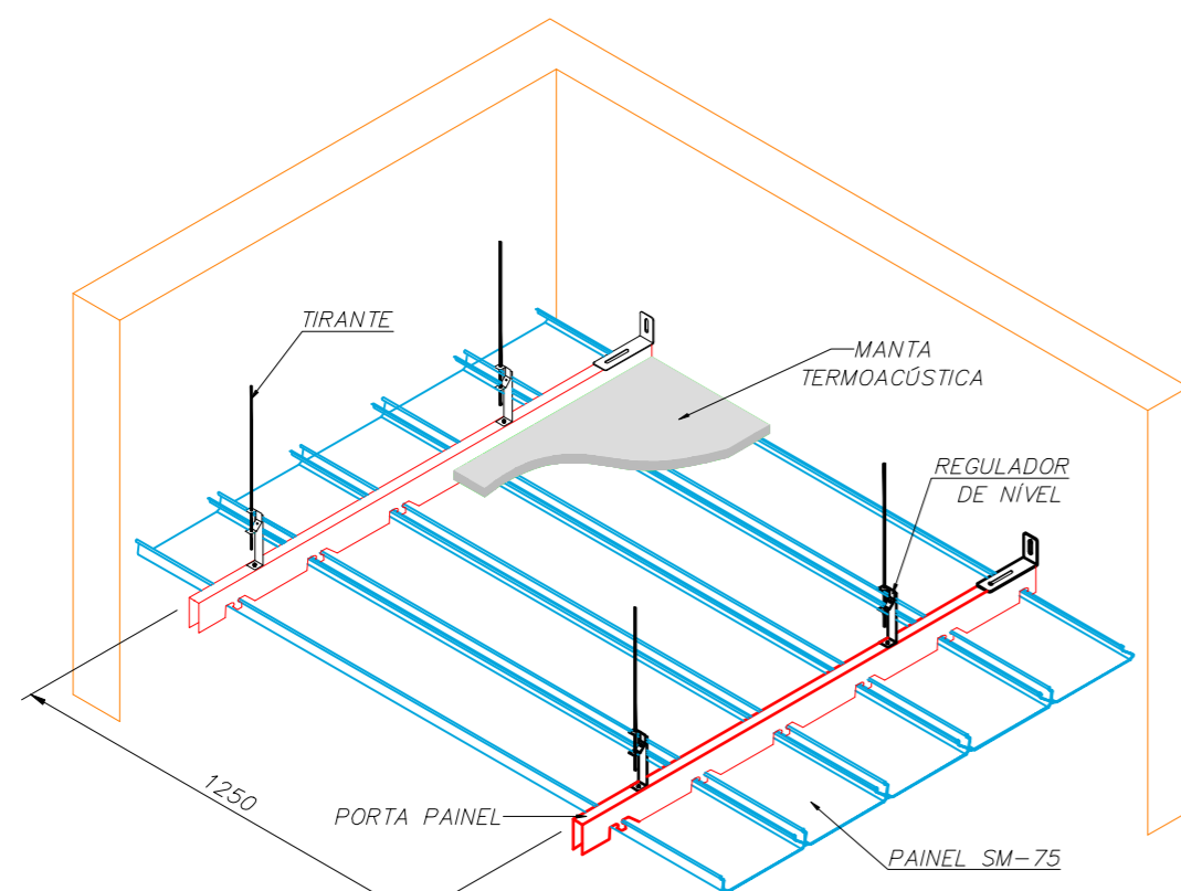
PERSPECTIVA FORRO SM-75 Escala: 5/8
