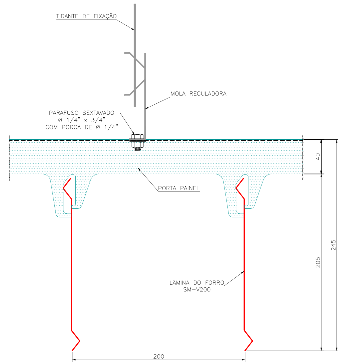
FORRO LINEAR SM-V200 ESCALA: 1:2
