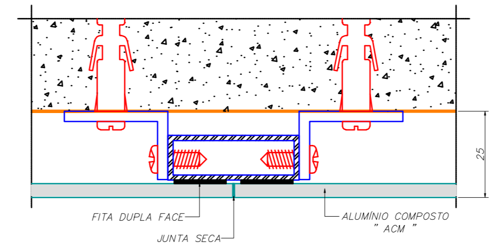
DETALHE TÍPICO DE JUNTA SECA
