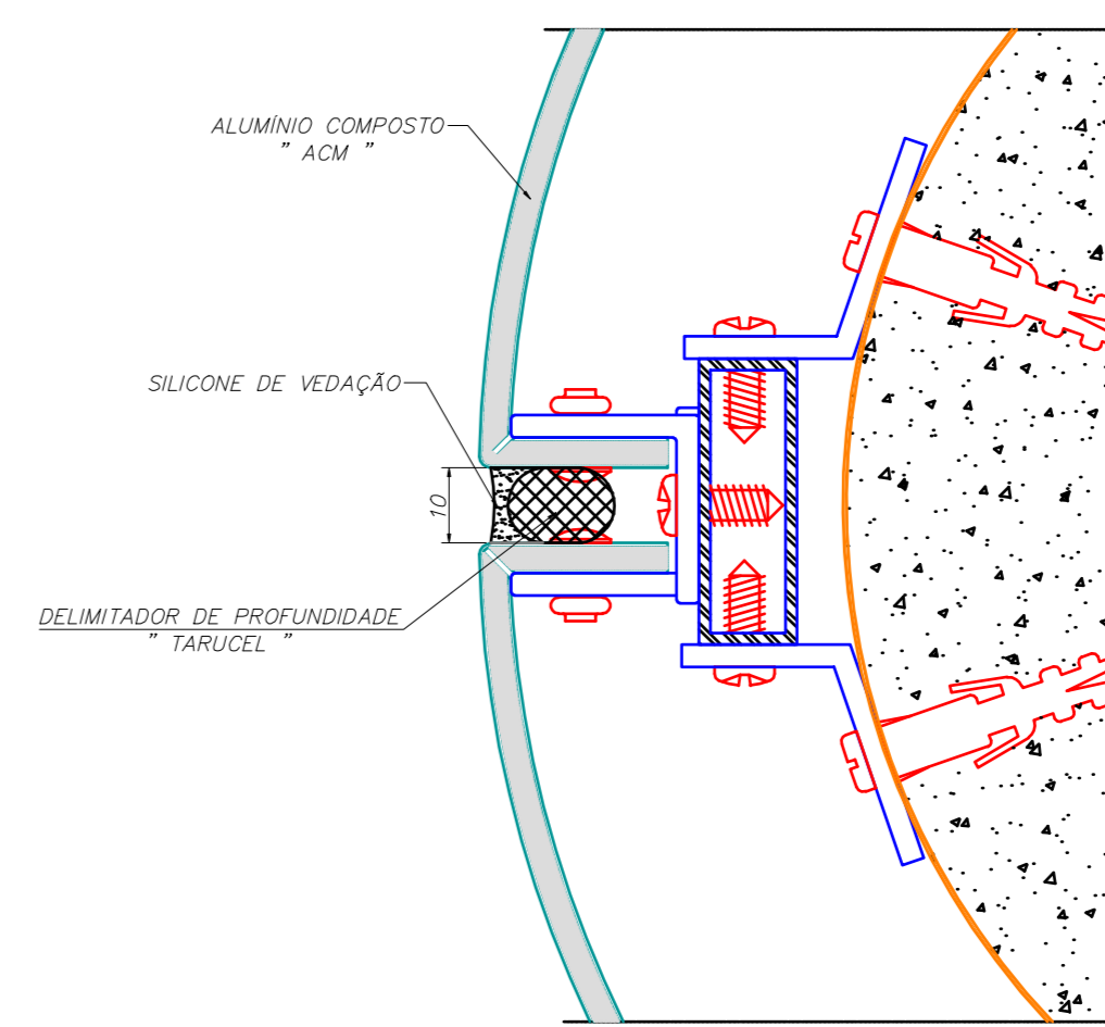
DETALHE DE CHAPA CALANDRADA
