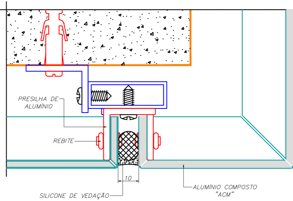
DETALHE DE CANTO
