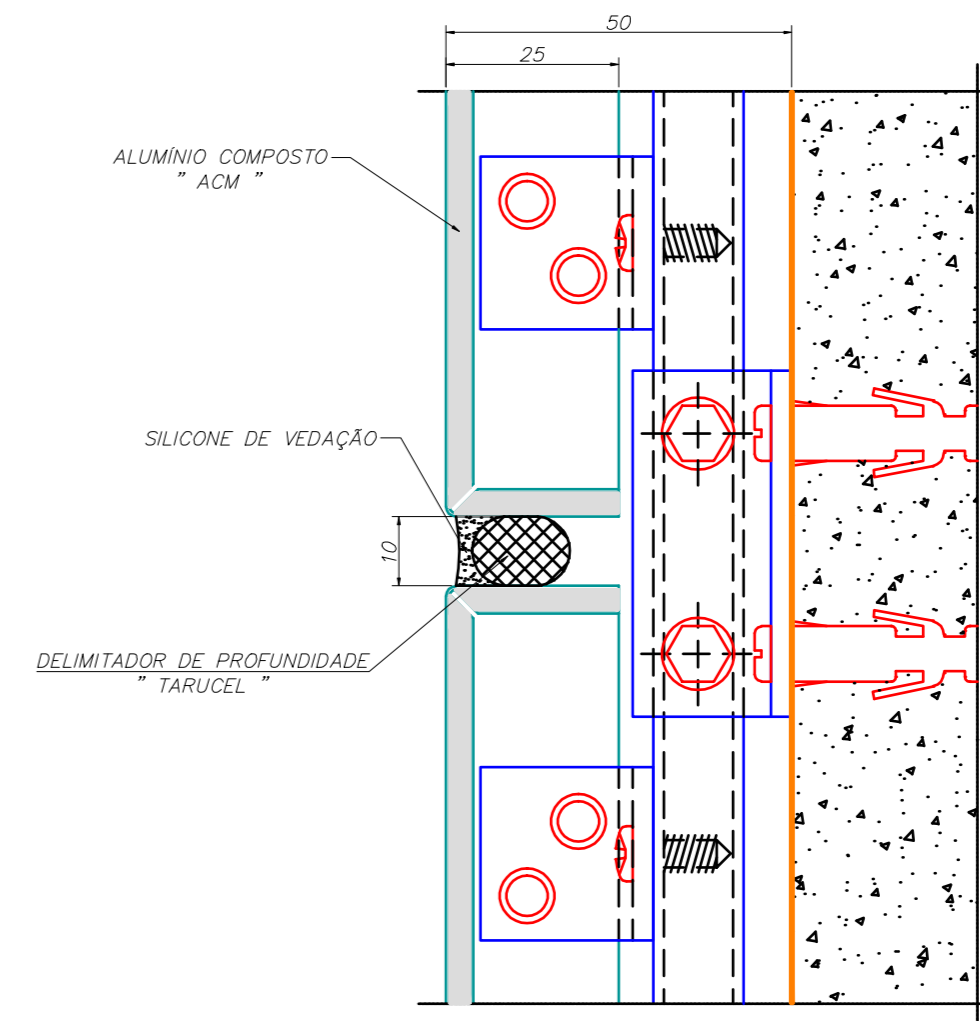
DETALHE TÍPICO DE JUNTA HORIZONTAL
