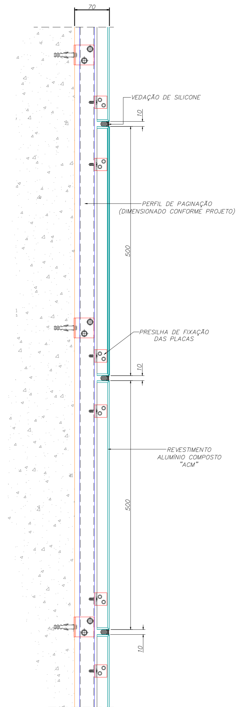
CORTE TÍPICO
