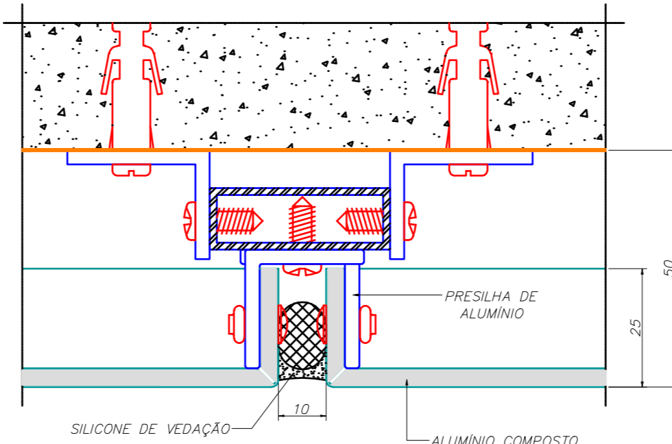
DETALHE TÍPICO DE JUNTA VERTICAL
