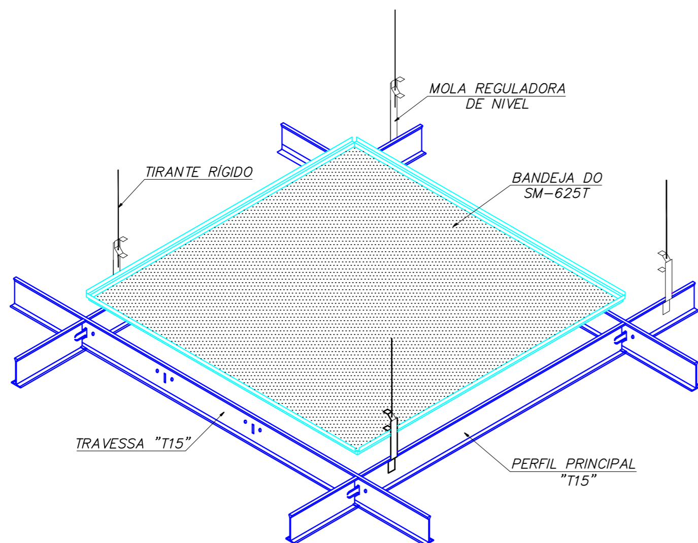
PERSPECTIVA MONTAGEM SM-625T Escala: S/E
