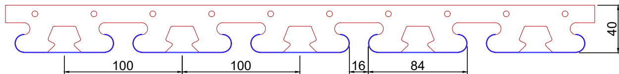
CORTE TÍPICO DO SM-M100 (SEM FLUSH)
