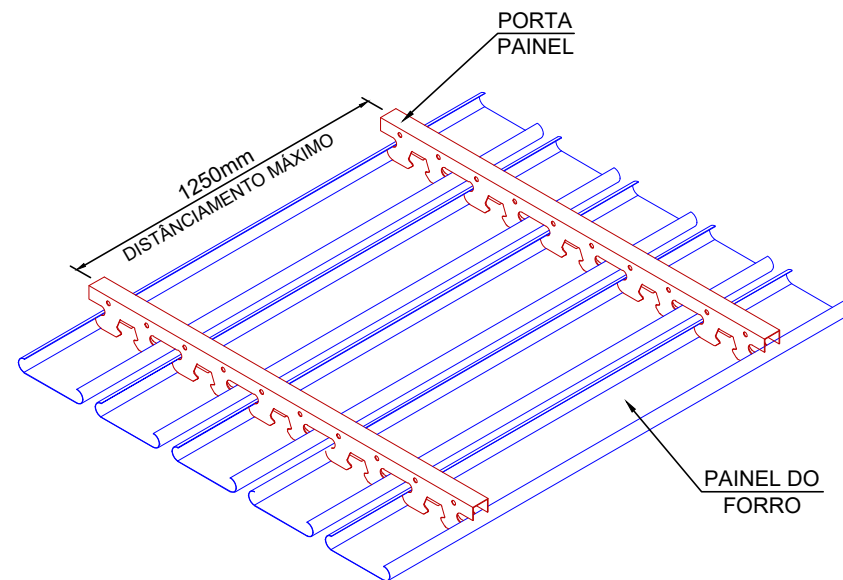
PERSPECTIVA DO FORRO
