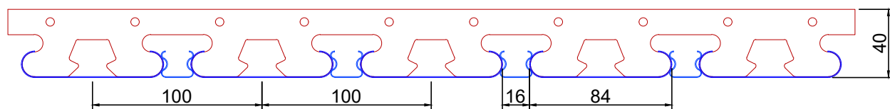
CORTE TÍPICO DO SM-M100 (COM FLUSH)
